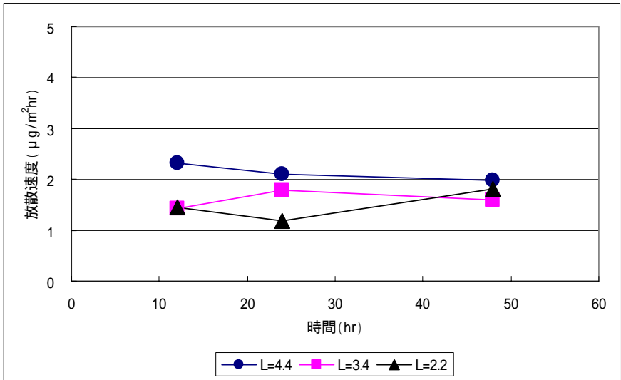
図 3-24 . 式から計算した放散速度 (静置)
