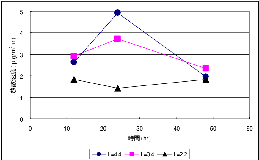
図 3-25 . 式から計算した放散速度 (攪拌)
