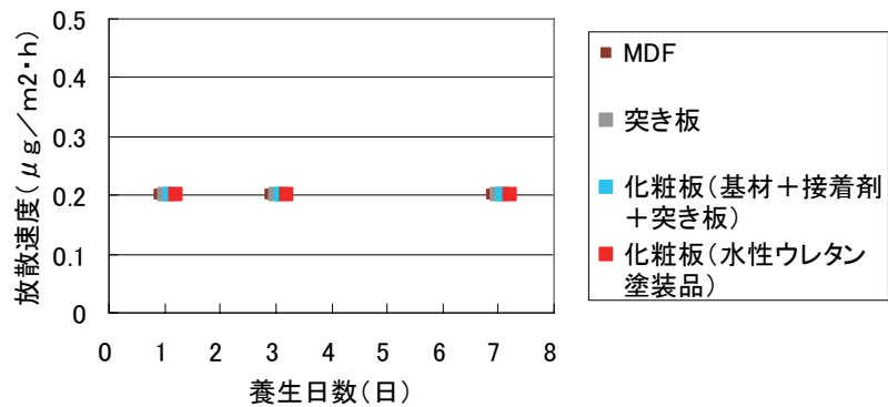
図 2-3 2 キシレンの放散 (縦軸 0 \sim 0.5 \mu\text{g} / \text{m}^2 \cdot \text{h} 表示)
