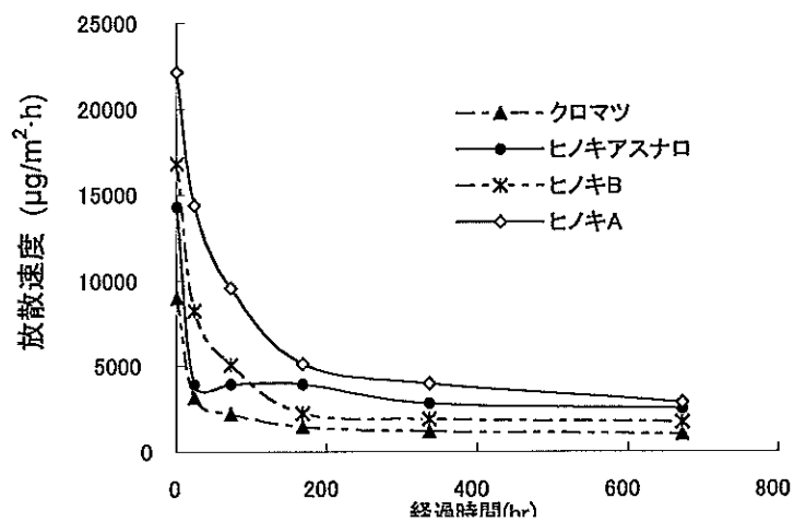
図 3-2 針葉樹材の TVOC(放散速度、トルエン換算)経時変化 (実験開始後 168 時間経過後 A: 100 \mu\text{g}/\text{m}^2\cdot\text{h} 未満、B(100 以上 1000 \mu\text{g}/\text{m}^2\cdot\text{h} 未満)、 C( 1000 以上 5000 \mu\text{g}/\text{m}^2\cdot\text{h} 未満))
