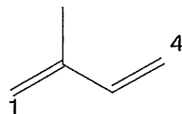
図 3-5 イソプレン単位
