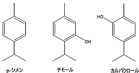
図 3-4 芳香族骨格を有するモノテルペン類
