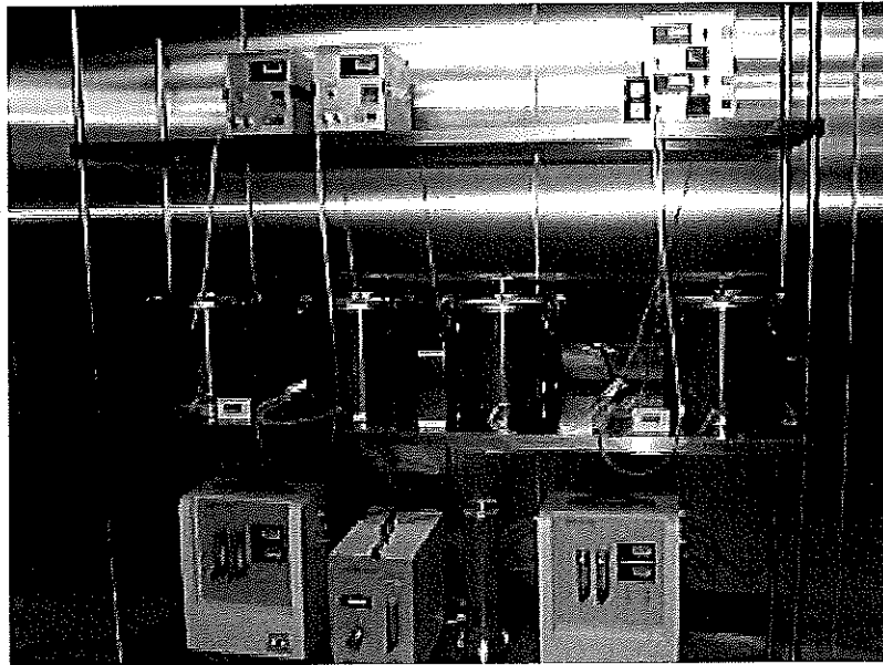
写真 6 - 1 小形チャンバーシステム
